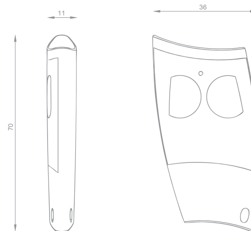
Dimensiones (mm)
