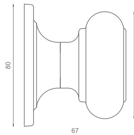
Dimensiones (mm)
