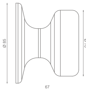
Dimensiones (mm)
