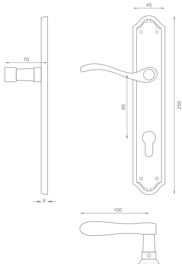
Dimensiones (mm)
