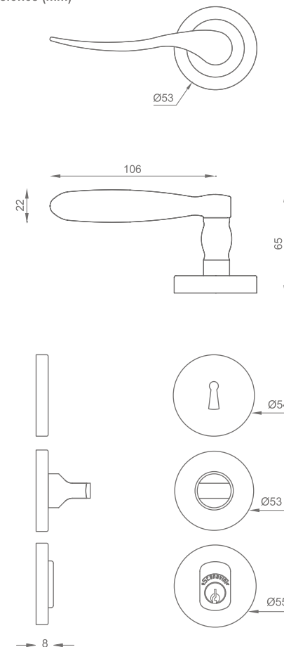
Dimensiones (mm)
