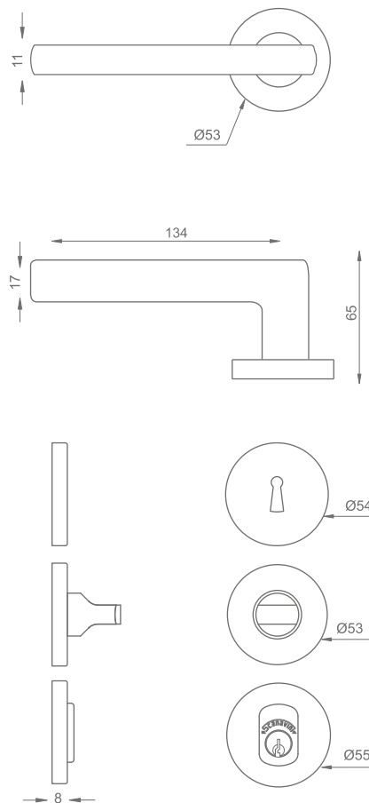
Dimensiones (mm)
