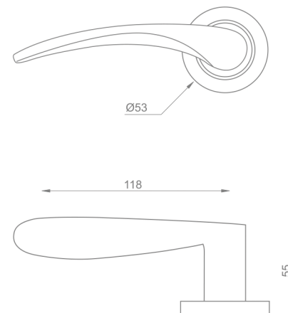
Dimensiones (mm)
