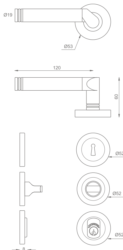
Dimensiones (mm)
