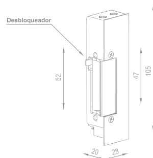
Dimensiones (mm)
