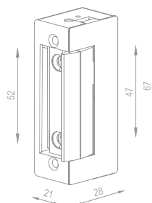
Dimensiones (mm)
