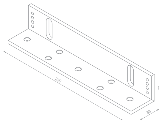
Dimensiones (mm)
