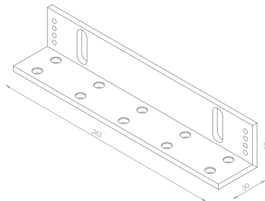
Dimensiones (mm)
