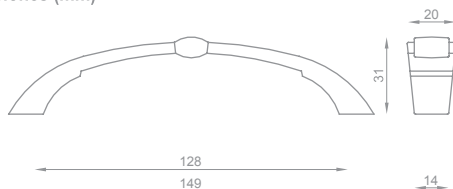
Dimensiones (mm)
