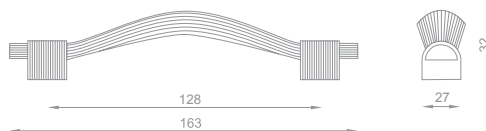
Dimensiones (mm)
