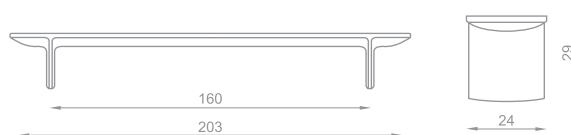
Dimensiones (mm)
